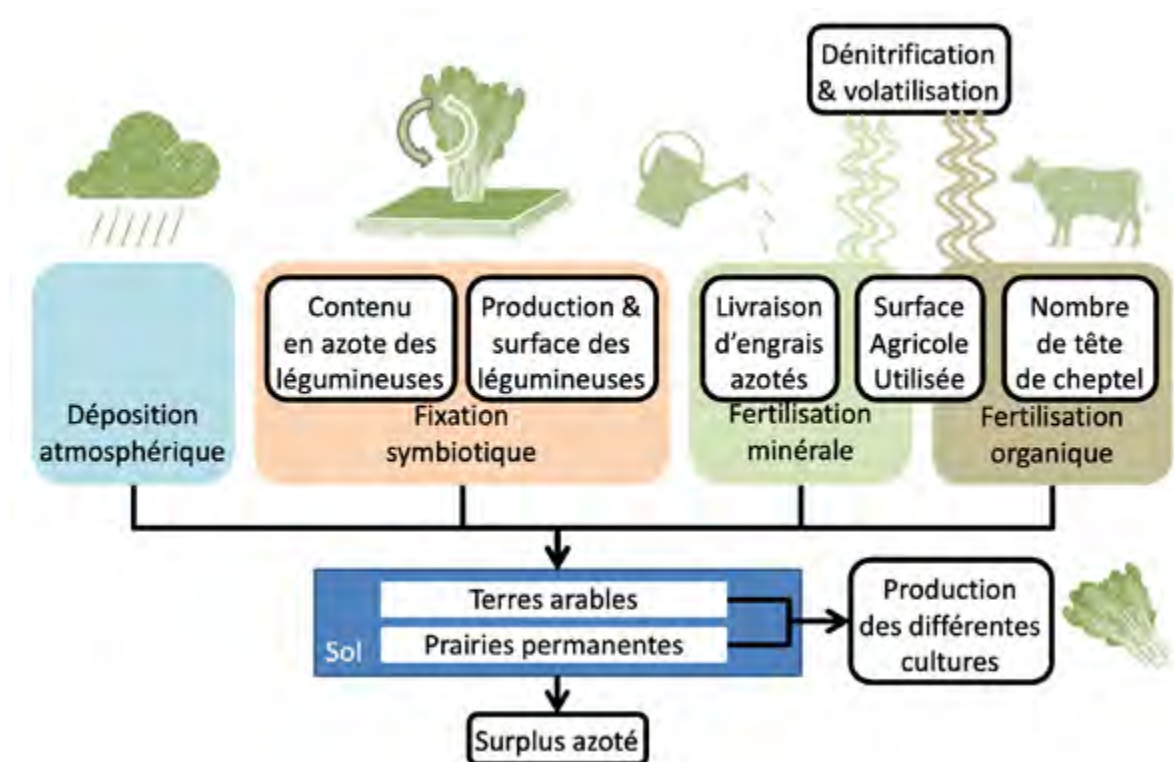
Figure 34 : Modèle CASSIS_N pour estimer la pression azotée diffuse
