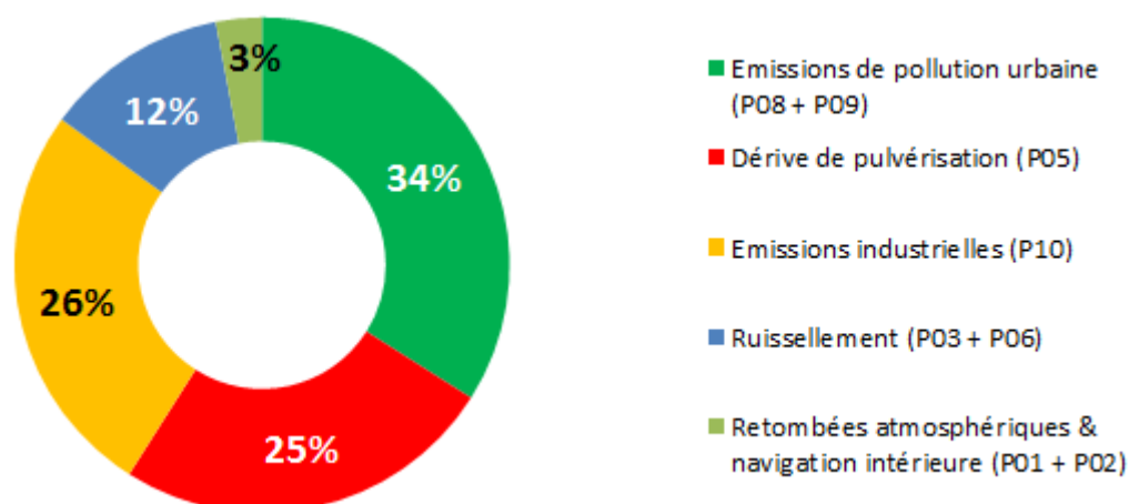
Figure 14 : Origine des substances dangereuses & déclassant les eaux
